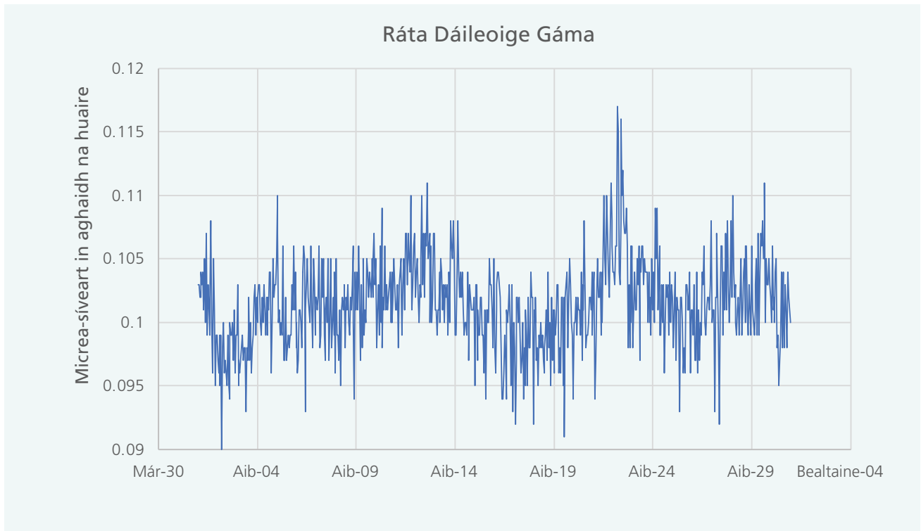
Fíor 19. Monatóireacht ar an Ráta Dáileoige Gáma Comhthimpeallach ag Dún Dealgan, Co. Lú
